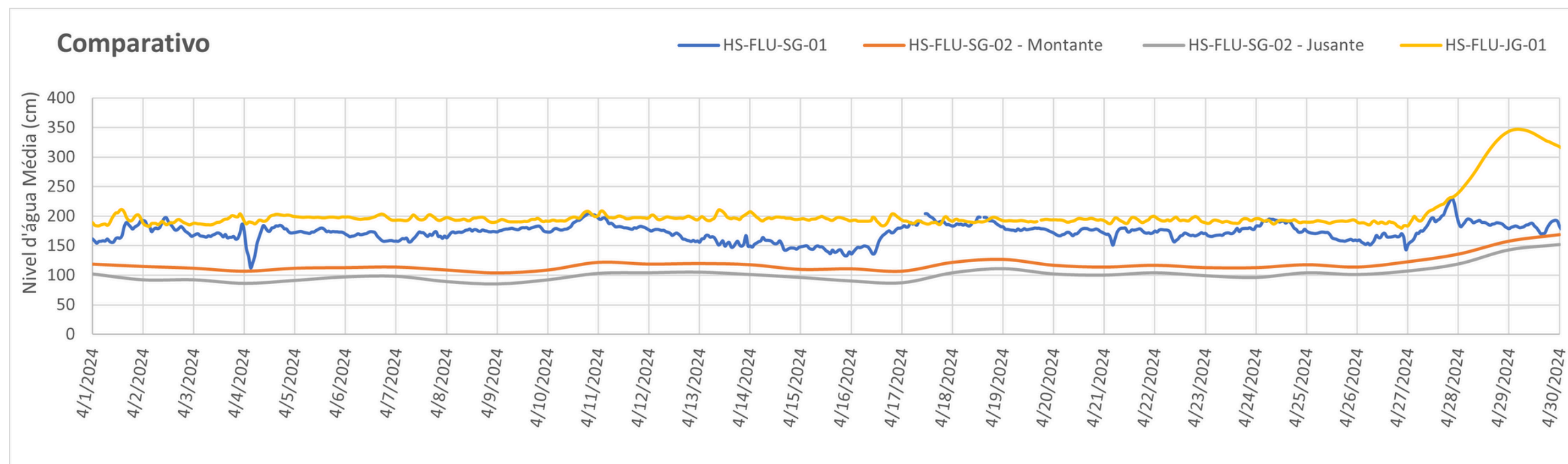
Figura 5 - Nível d'água médio (cm) comparativo nas Estações supracitadas: Estação Santa Santa Isabel do Sul (Azul) Estação Barragem do Canal São Gonçalo - Montante (Laranja) Estação Barragem do Canal São Gonçalo - Jusante (Cinza) Estação Jaguarão (Amarelo)
