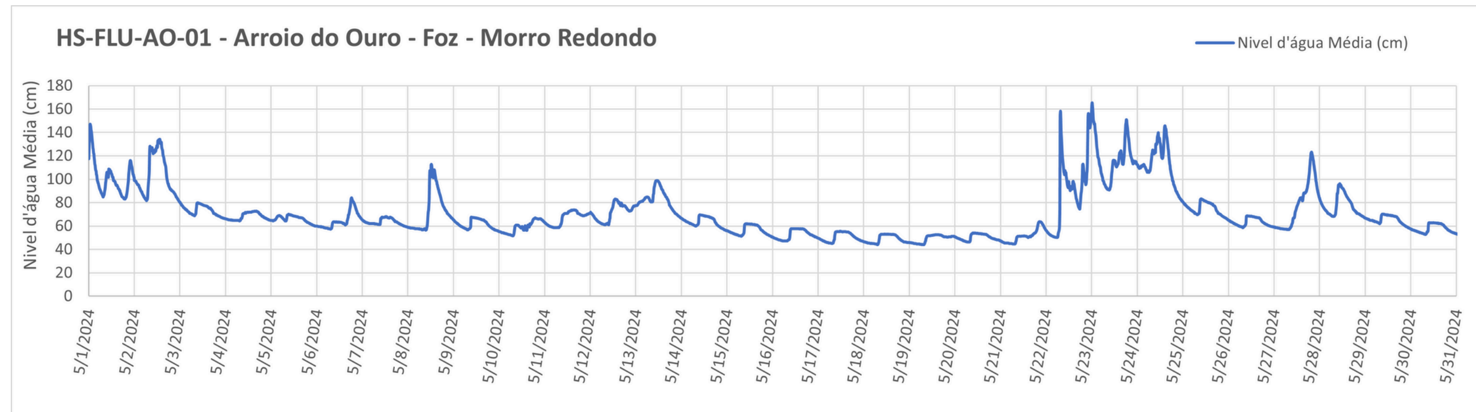
Figura 7 - Nível d'água médio (cm) na Estação o Arroio do Ouro (Foz).
