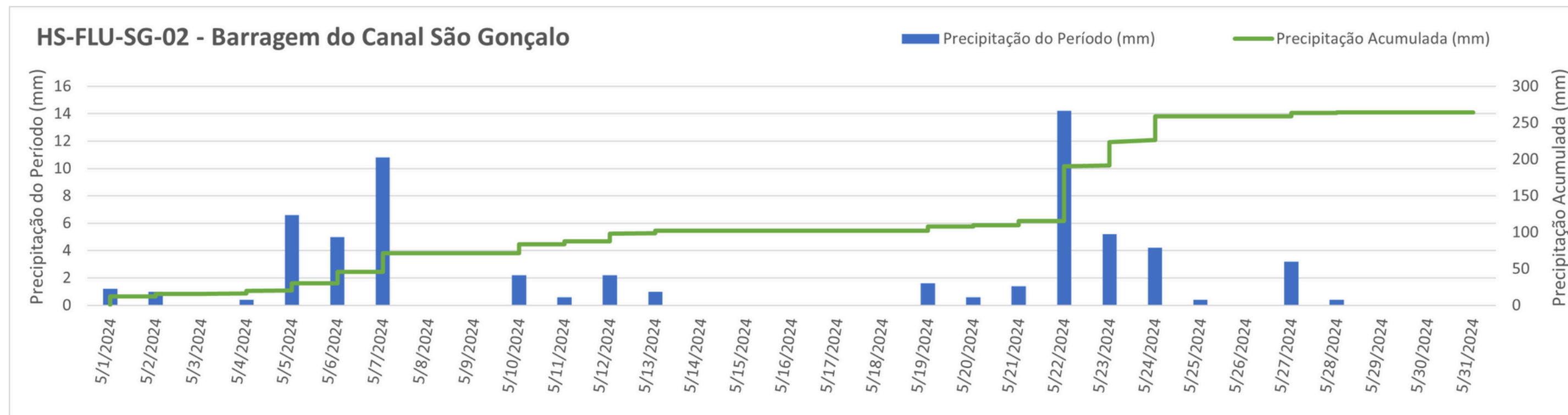
Figura 10 – Precipitação (mm) na Estação Barragem do Canal São Gonçalo.
