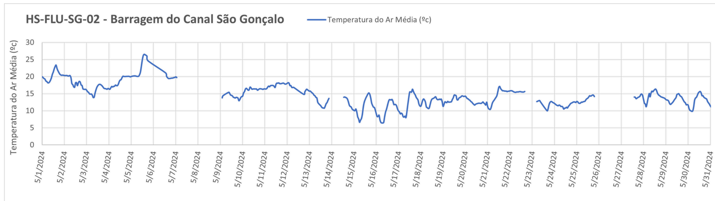
Figura 13- Temperatura média da Estação Barragem do Canal São Gonçalo.
